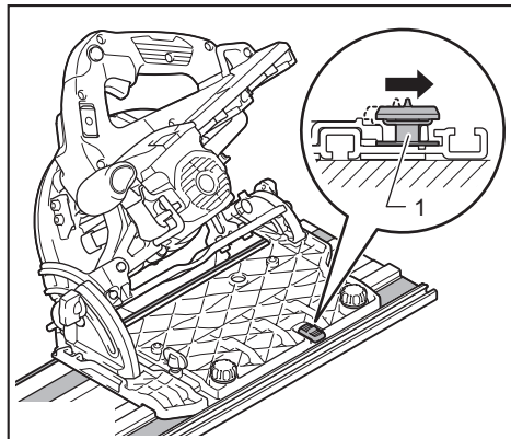
► 1. Levier coulissant
