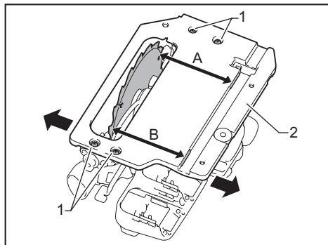
► 1. Vis 2. Base
