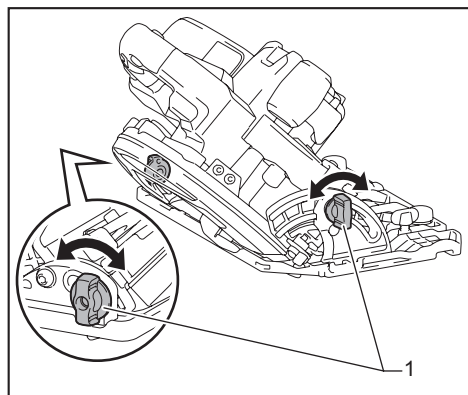
► 1. Clamping screw
